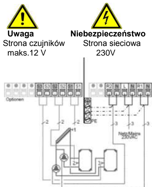
Rys. 3.2.11 " Solar z dwoma zasobnikami równoległymi-2 pompy"
